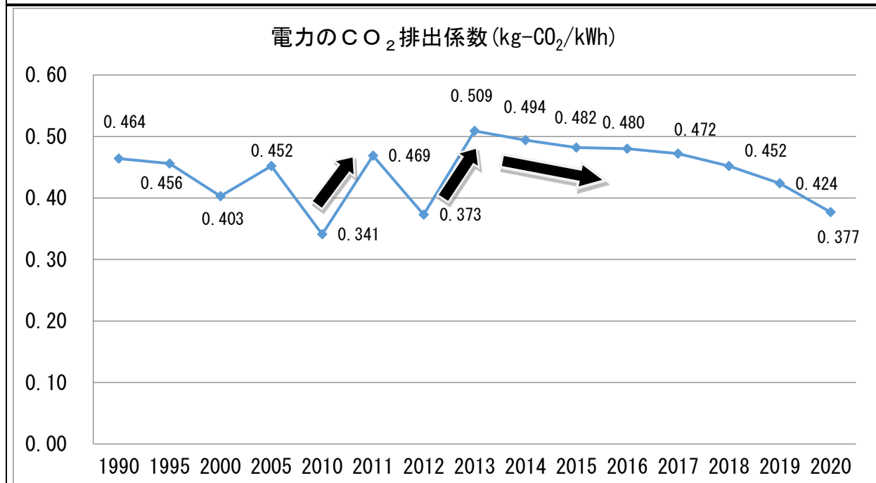
図2 中部電力株式会社のCO 2 排出係数の変遷
