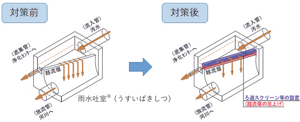
合流改善施設のイメージ (注)
